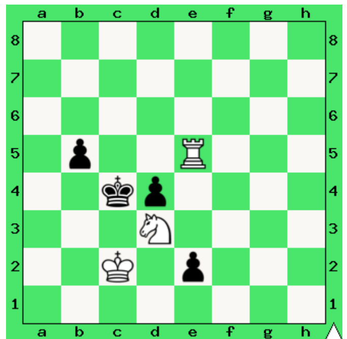
Zadanie 4. Mat w 1 posunięciu.
