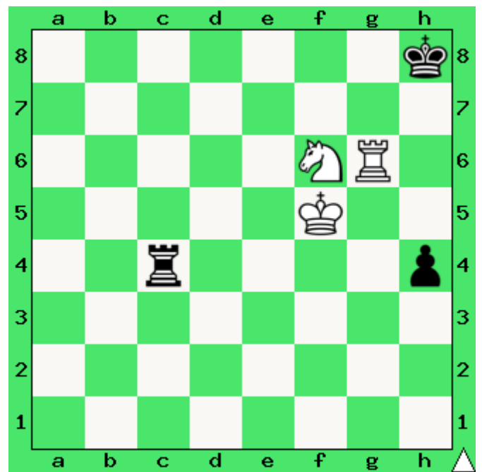
Zadanie 2. Mat w 1 posunięciu.
