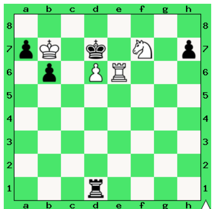
Zadanie 6. Mat w 1 posunięciu.
